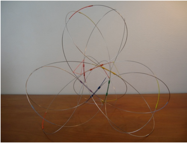
Représentation symbolique de la surface de Boy en trois dimensions
