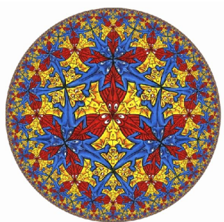
Jos Leys. Escher E 85
