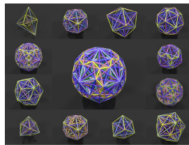
Francesco De Comite. Les polyèdres d'Archimède
