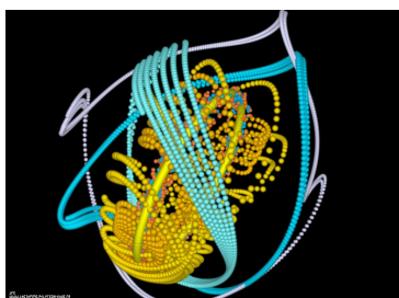
J.-F. Colonna. Trajectoires des planètes vues système solaire vues d'une planète virtuelle
