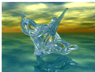
L. Bénard. Respiration silencieuses des solitons
