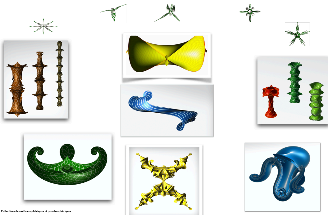
David Brander. Collections de surfaces sphériques et pseudo-sphériques
