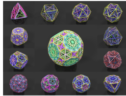
Francesco de Comite. Les polyèdres de Catalan
