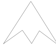
Fig.11: Hexagone d'indice 1
