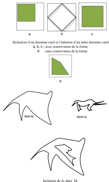
Fig.49: Exemples élémentaires
